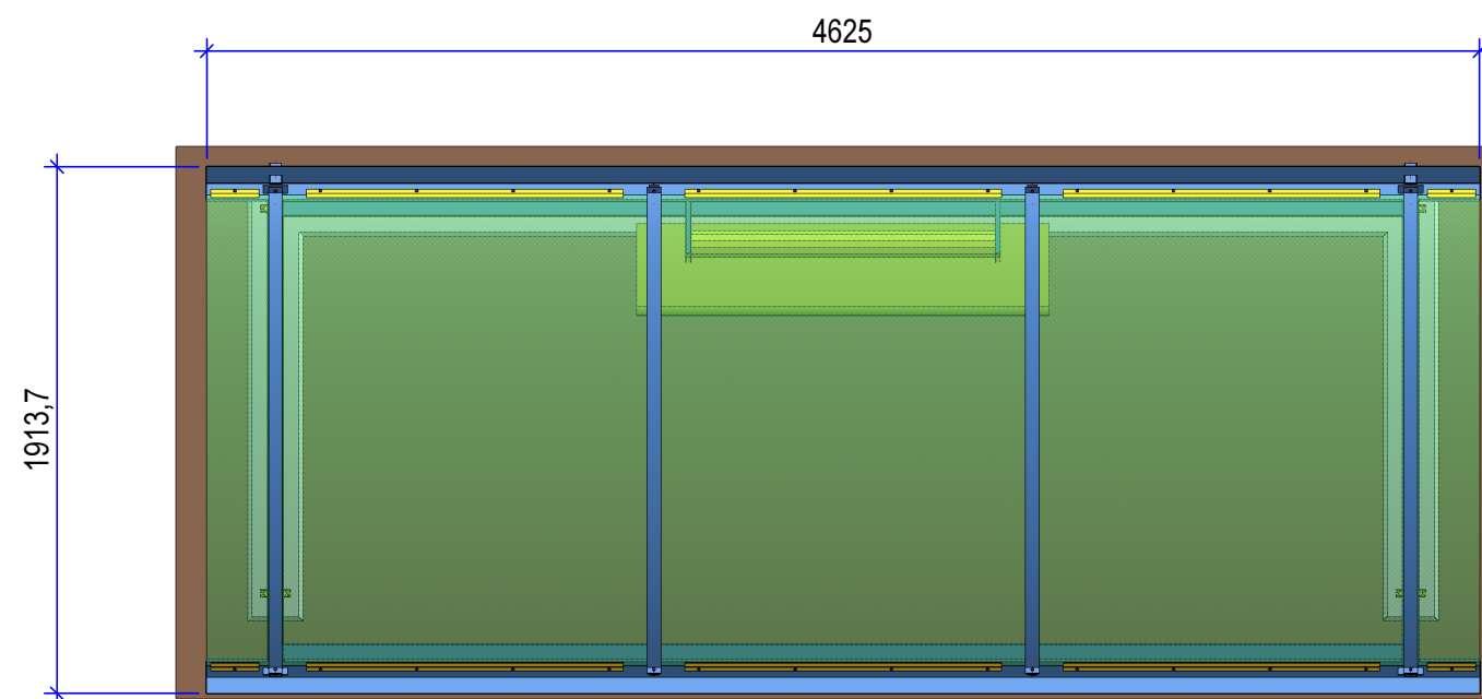
Grundriss
