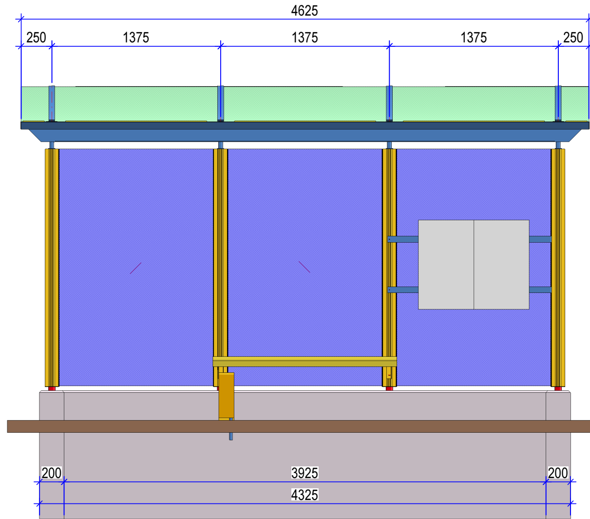
Ansicht
