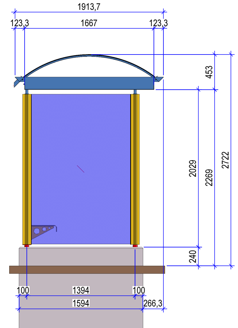
Seitenansicht
