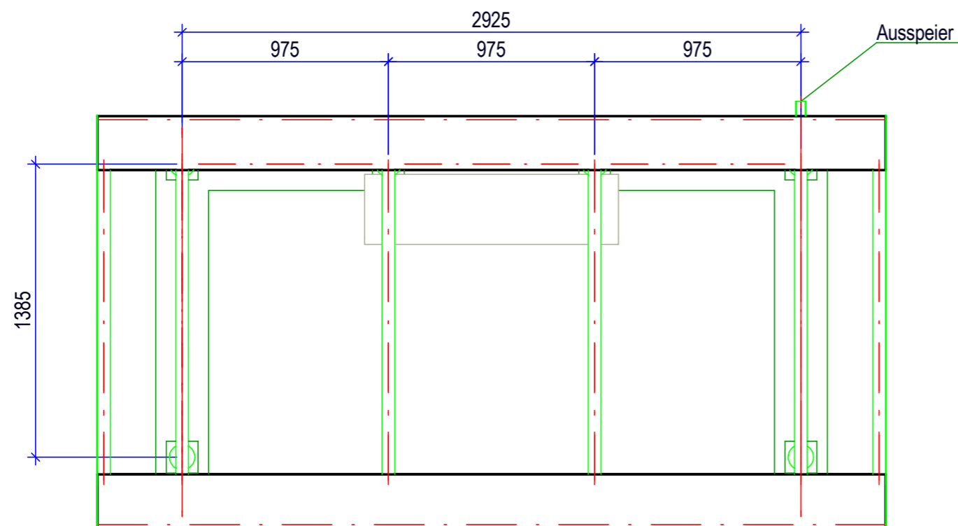
Grundriss
