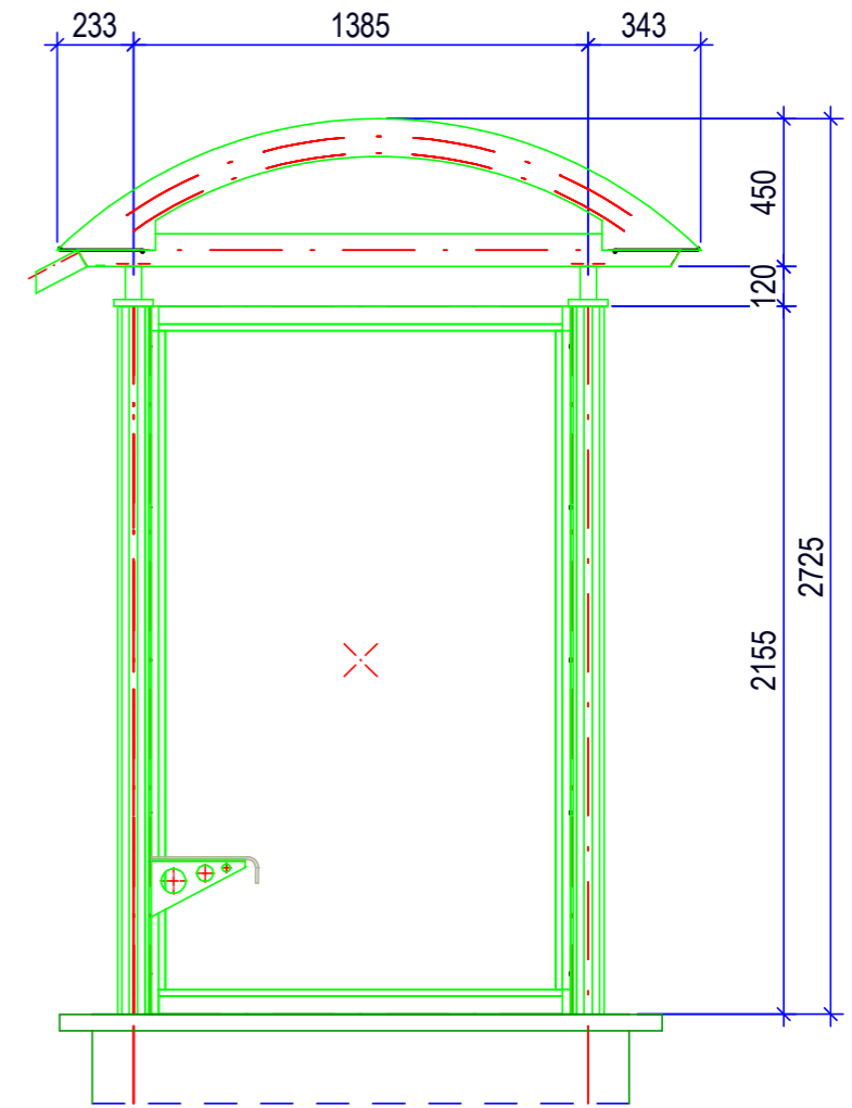
Seitenansicht
